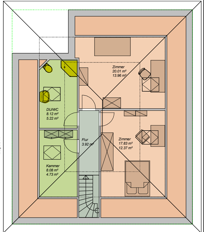
Grundriss Dachgeschoss
